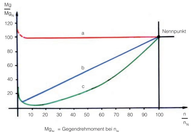
Abb. 2: Typische Drehmomentverläufe von Arbeitsmaschinen
