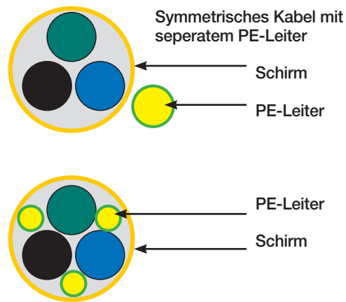
Abb. 6: Ausführungen mehradriger symmetrischer Motorkabel
