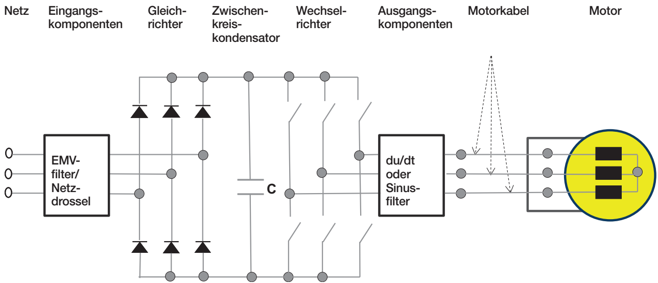
Abb. 1: Hauptkomponenten eines Antriebssystems
